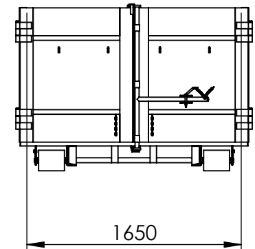
DRZWI
