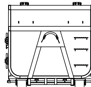
PRZOD
