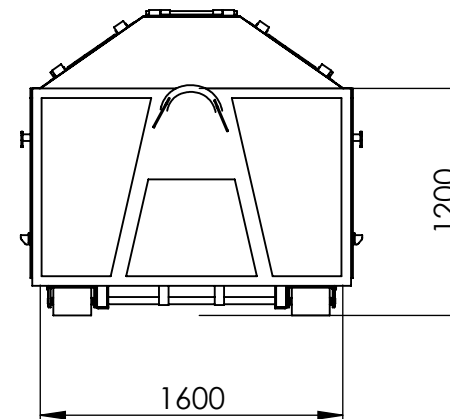
PRZÓD — HAK
