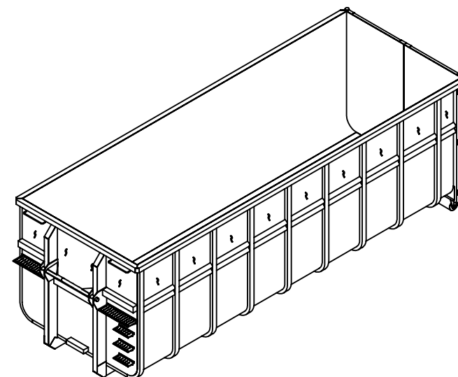
AKSONOMETRIA 1:75
