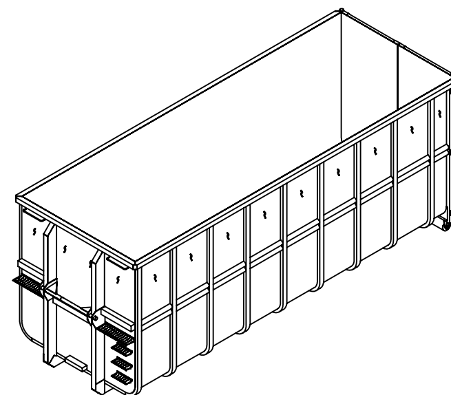
AKSONOMETRIA 1:75
