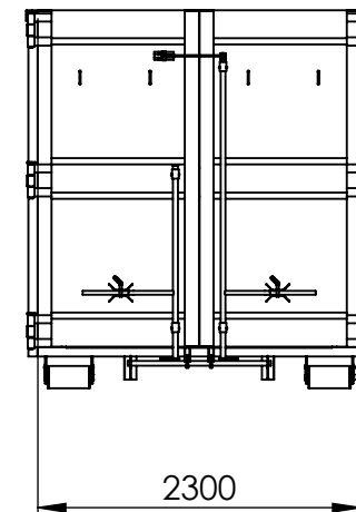
DRZWI
