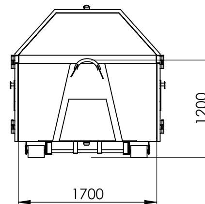
TYŁ — DRZWI
